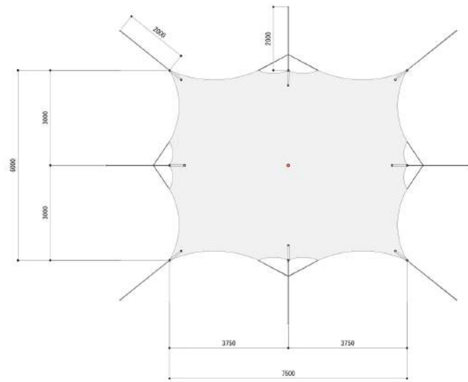
plan [scale: 1/100]
